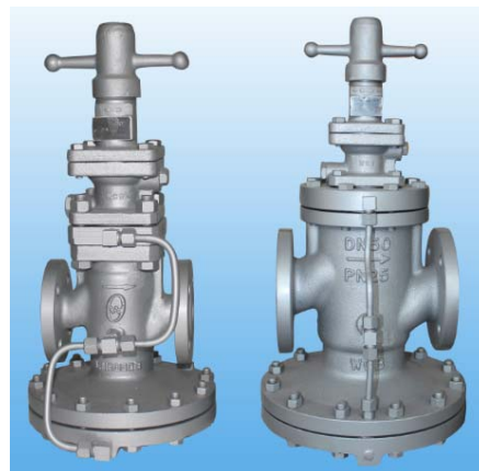
口径: DN15-25 口径: DN32-100
